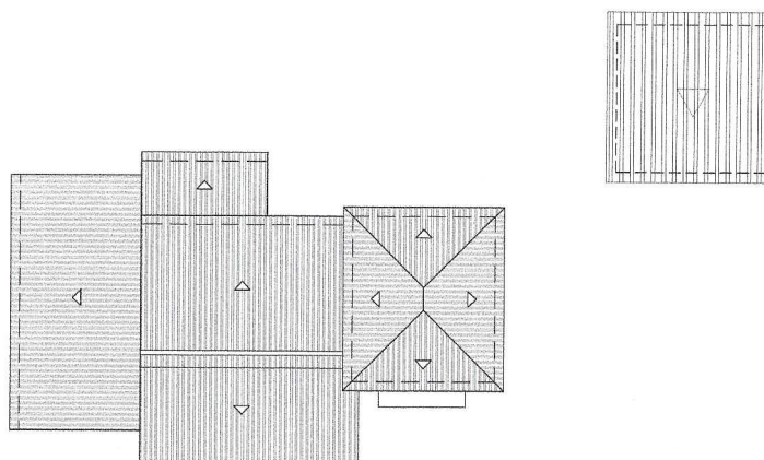
PLANTA CUBIERTA 1:100
