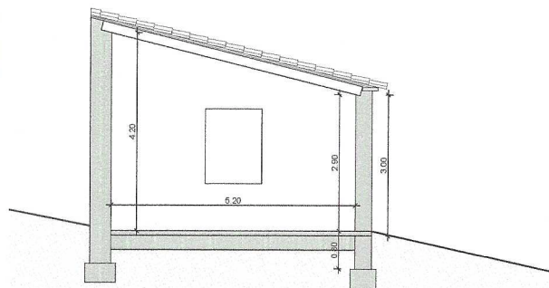
SECCIÓN GARAJE
