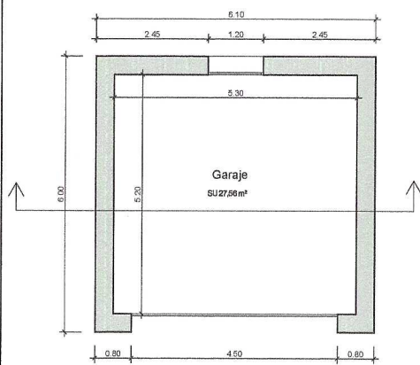
PLANTA GARAJE
