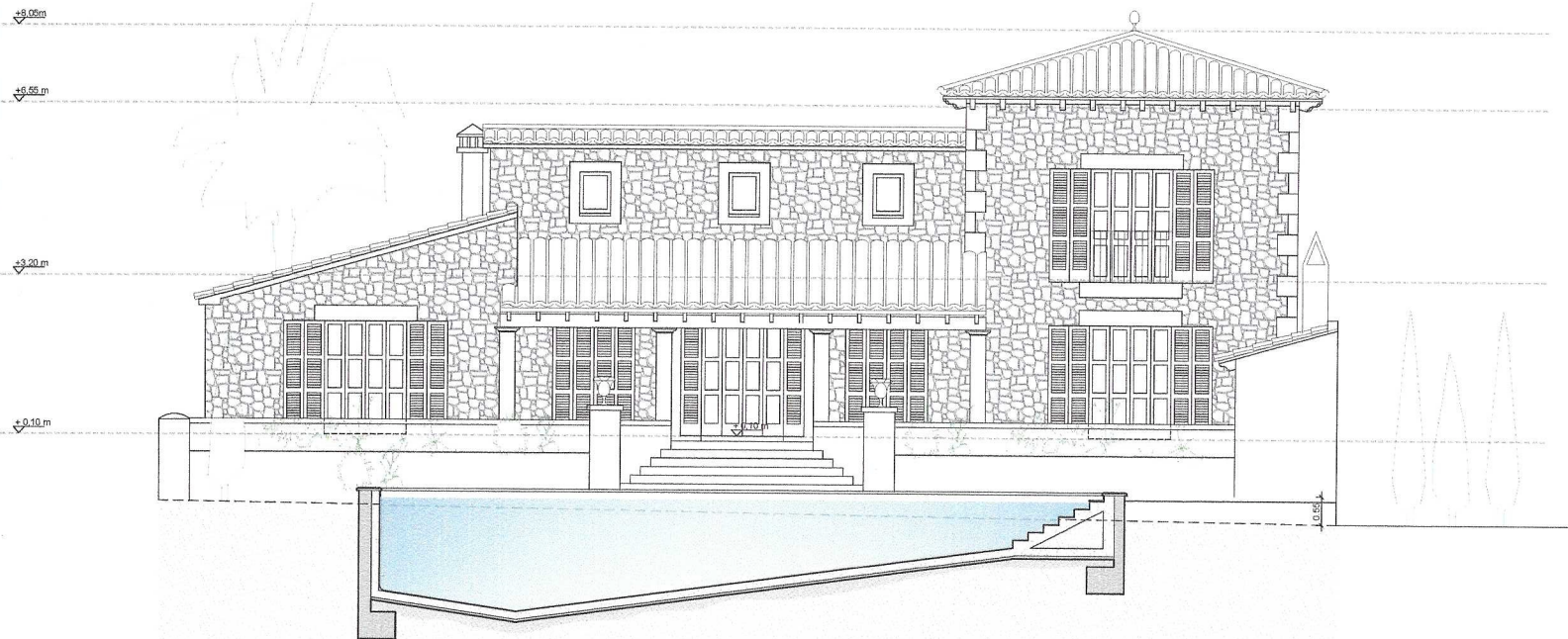
ALZADO PONIENT
