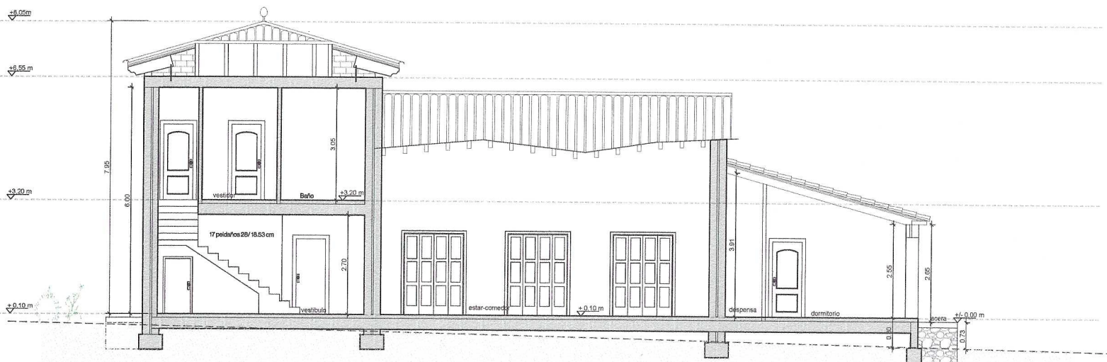
SECCION TRANSVERSAL
